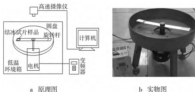
图 1 实验装置
