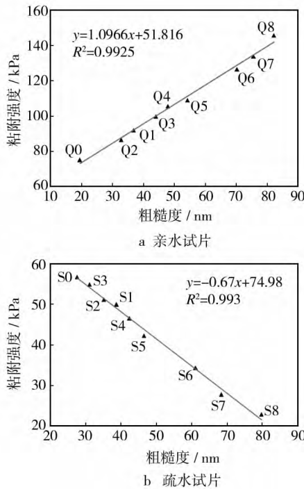
图 3 冰粘附强度与表面粗糙度的关系
