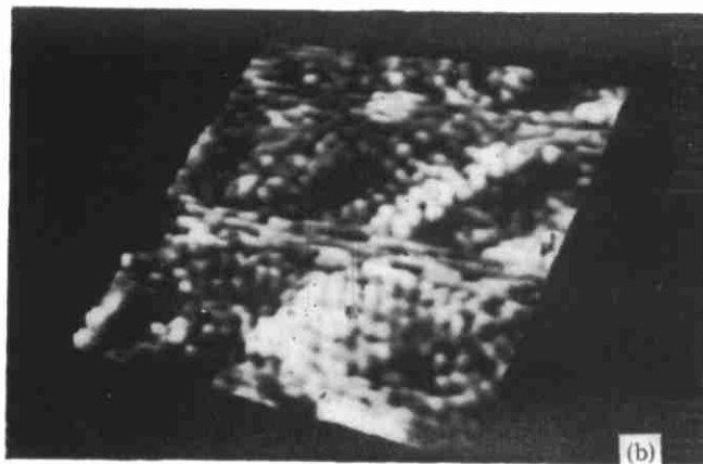
(b) 相应的平面图 ( 41 \text{ \AA} \times 48.8 \text{ \AA} )
