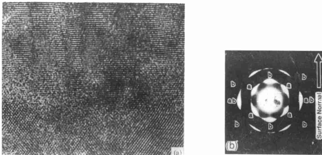
图1 nc-Si:H 膜 HREM 照片
